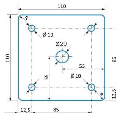
príruba KPS
